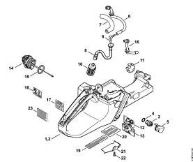
Těleso nádrže
