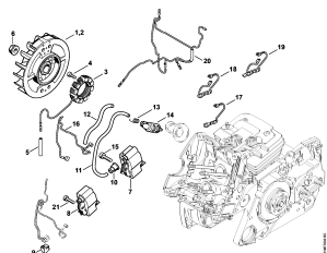
Zapalování, kabelový svazek
