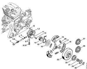
Olejové čerpado, spojka
