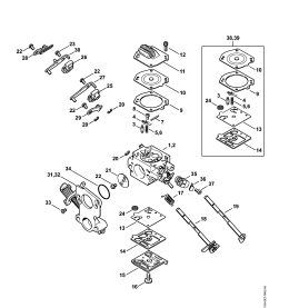
Karburátor HD-49B, HD-47
