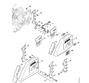
Zařízení pro napínání řetězu
