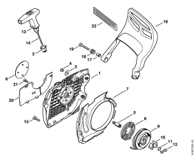
Startovací zařízení
