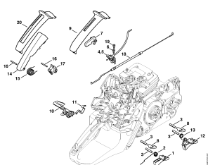
Ovládání plynu
