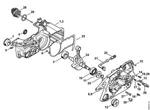
Kliková skříň
