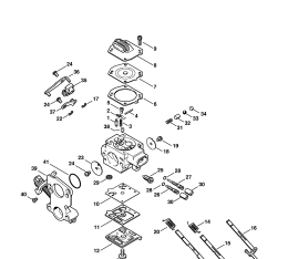
Karburátor HD-41
