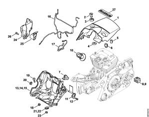
Kryt, skříň/těleso
